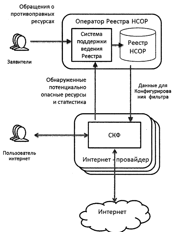
Рисунок 6. Принцип контроля доступа через Реестр NSCOP
